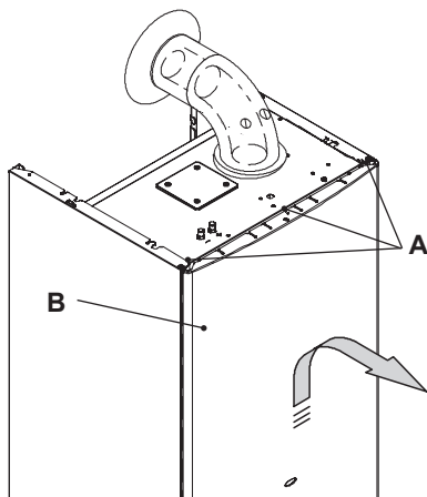
Fig. 9.1 Pannelli laterali
