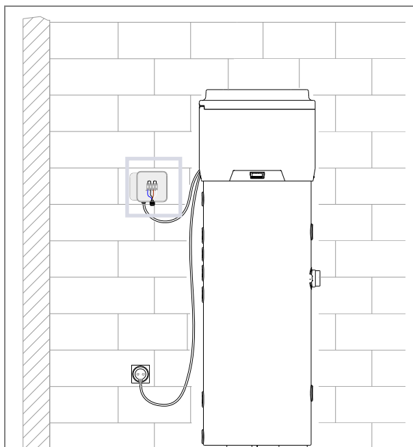
Fig. 11 - Esempio connessione remota
