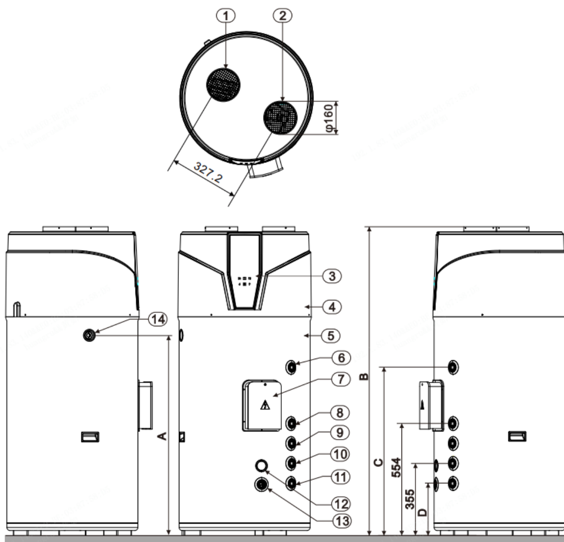
Fig. 3.1 - Disposizione e dimensioni NEOS TOP 200S
