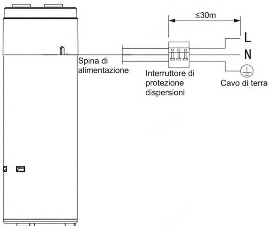
Fig. 8 – collegamento a terra
