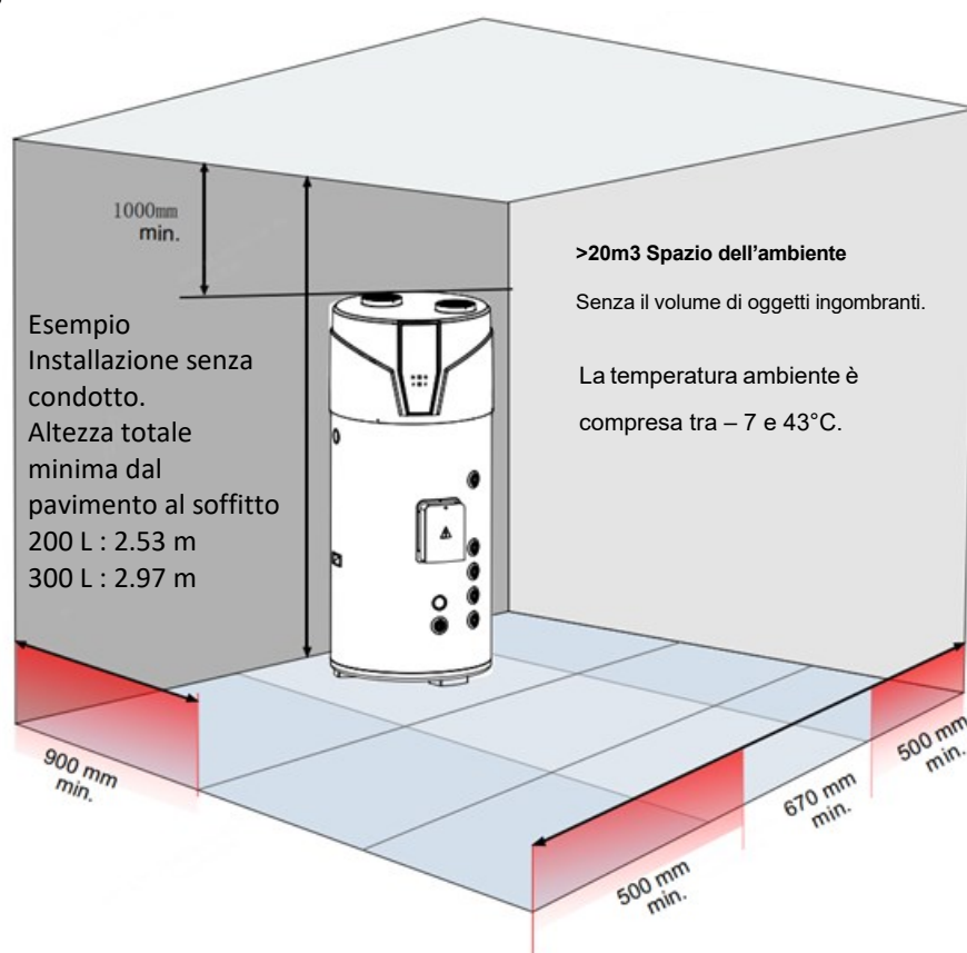
Fig.4 Spazio consigliato per installazione e manutenzione
