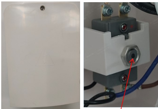
Pulsante di ripristino nero del termostato
