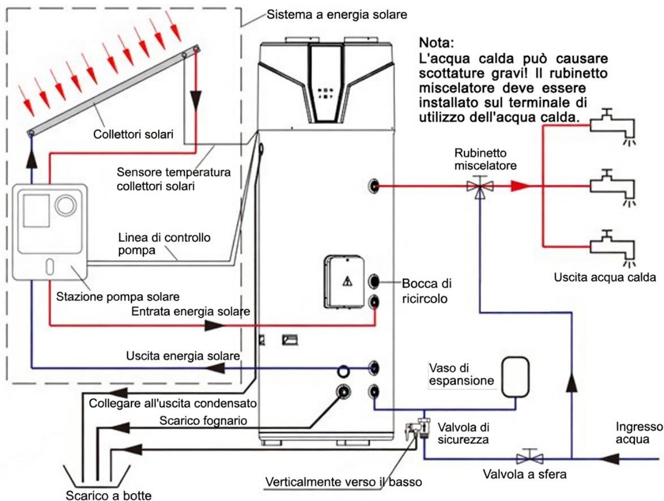
Fig. 6 – Connessioni idrauliche
