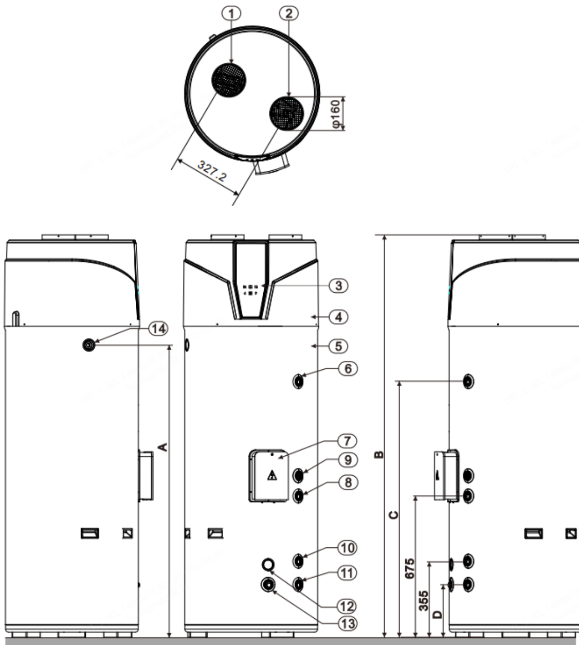
Fig. 3.1 - Disposizione e dimensioni NEOS TOP 300S
